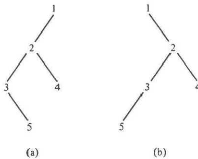
Fig. 3.19. Dos árboles binarios.
