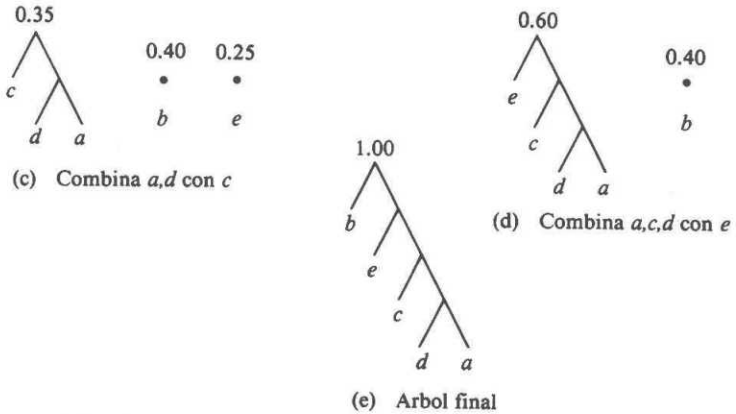
Fig. 3.24. Pasos para la construcción de un árbol de Huffman.
